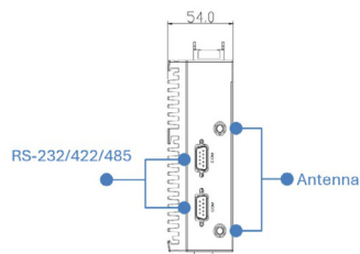
Top I/O
